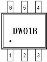
SOT23-6
